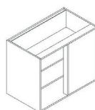
Meuble Bas angle droit porte Ht 800 Prof 580
